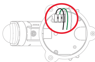
Cámara con proyector, conector inferior de 3 cables
