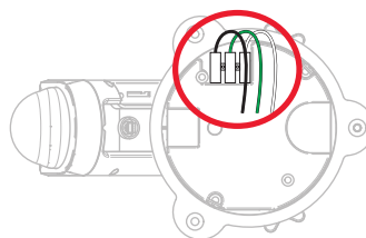
Caméra avec projecteurs, connecteur inférieur à 3 fils
