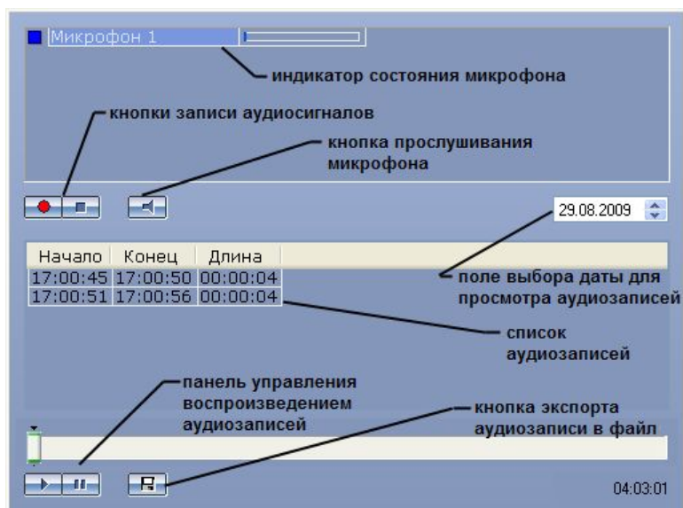
Рис. 5—3 Пример стандартного интерфейса Аудиопроигрывателя
